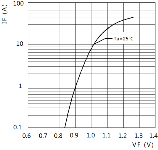
图 4. 典型正向特性
